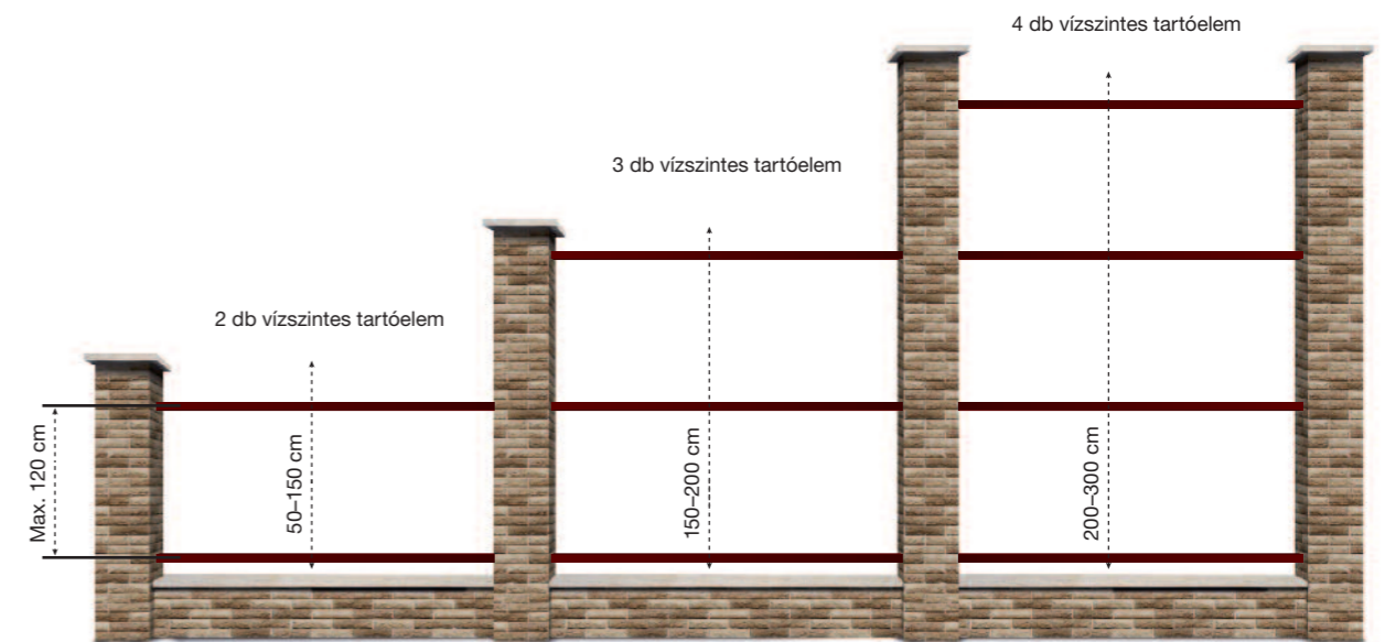
Kerítésszerkezet előkészítése függőleges kerítéselemek fogadására
