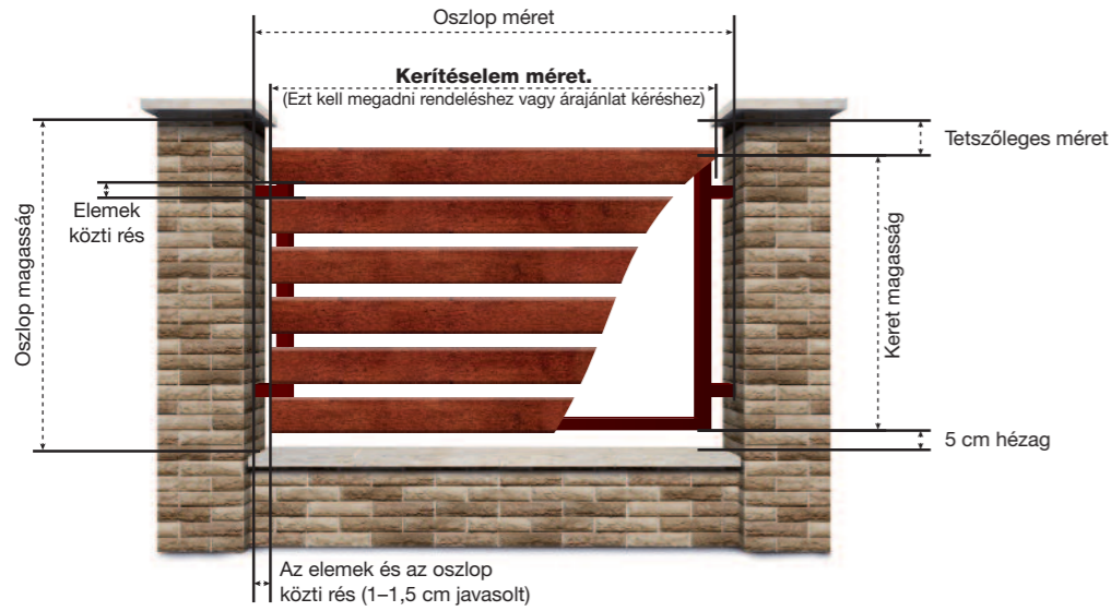
Kerítésszerkezet előkészítése vízszintes kerítéselemek fogadására
