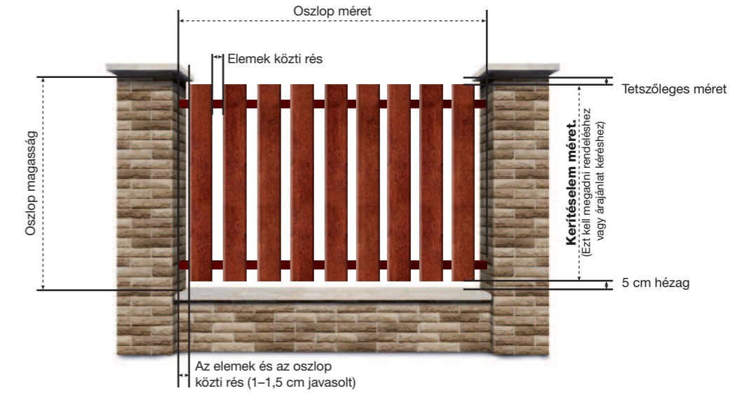
Kerítésszerkezet előkészítése függőleges kerítéselemek fogadására
